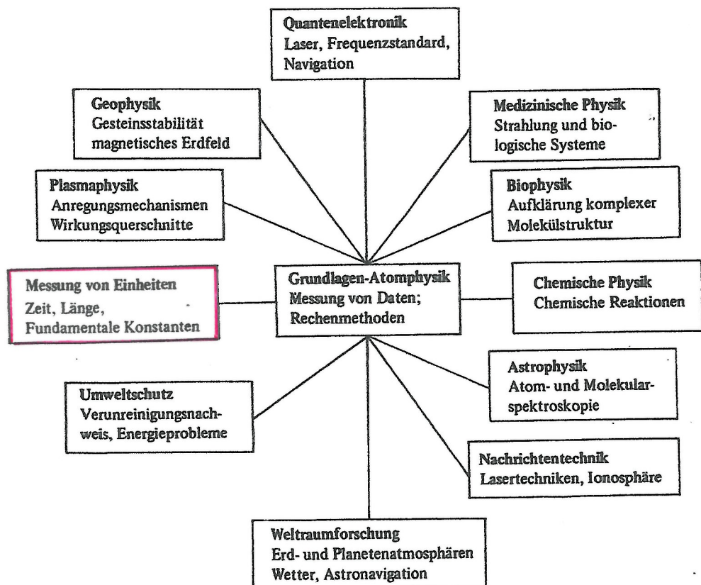
Fig. 2 Beziehung der Atomphysik zu anderen Wissenschaftsbereichen (in Anlehnung an Physics in Perspective, s. Fig. 1)
