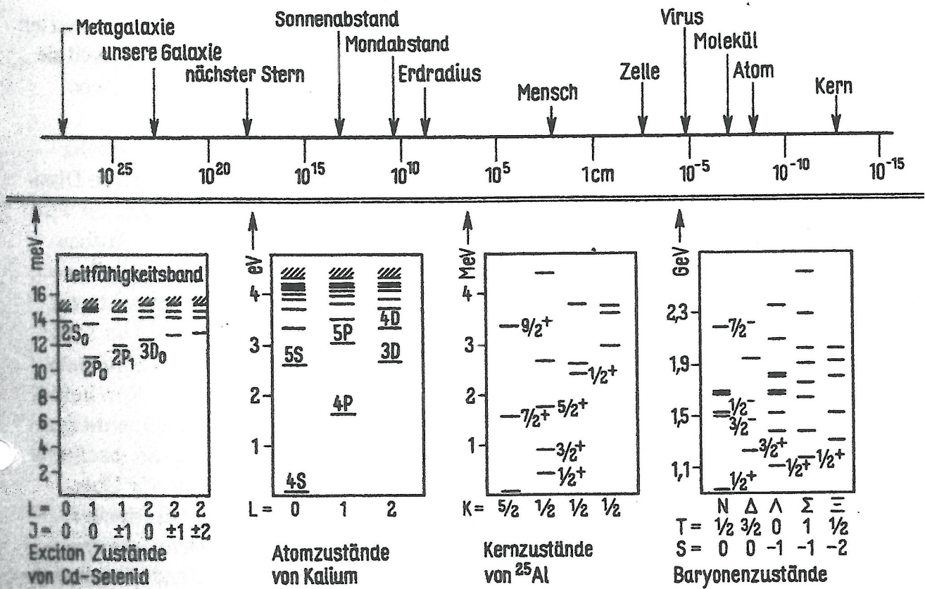
Fig. 1 Oben: Größenskala verschiedener Naturobjekte.
