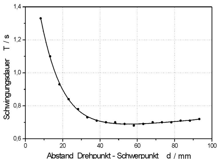
Abb. 4.2 Abhängigkeit der Schwingungsdauer T von der Pendellänge d .
