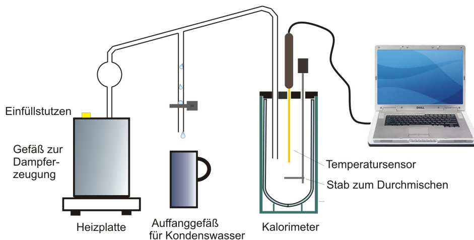
Abb. 3.1 Experimentelle Anordnung
