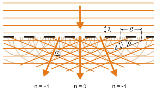
Abb. 2.1 Entstehung von Wellenfronten unterschiedlicher Ausbreitungsrichtung
